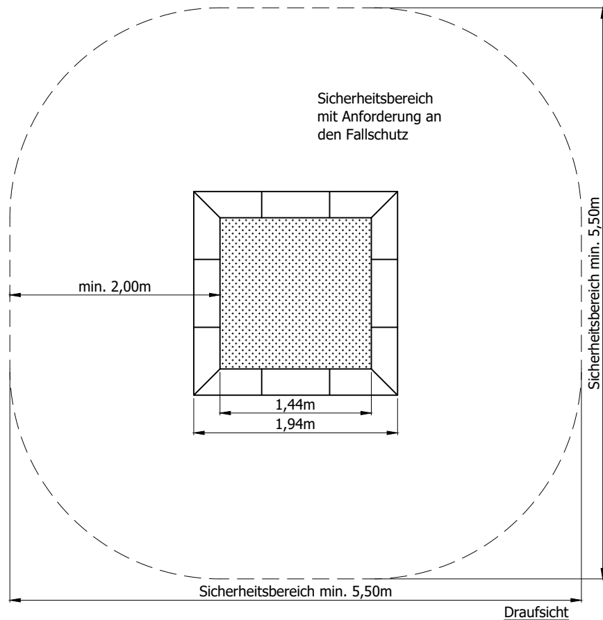
Draufsicht
