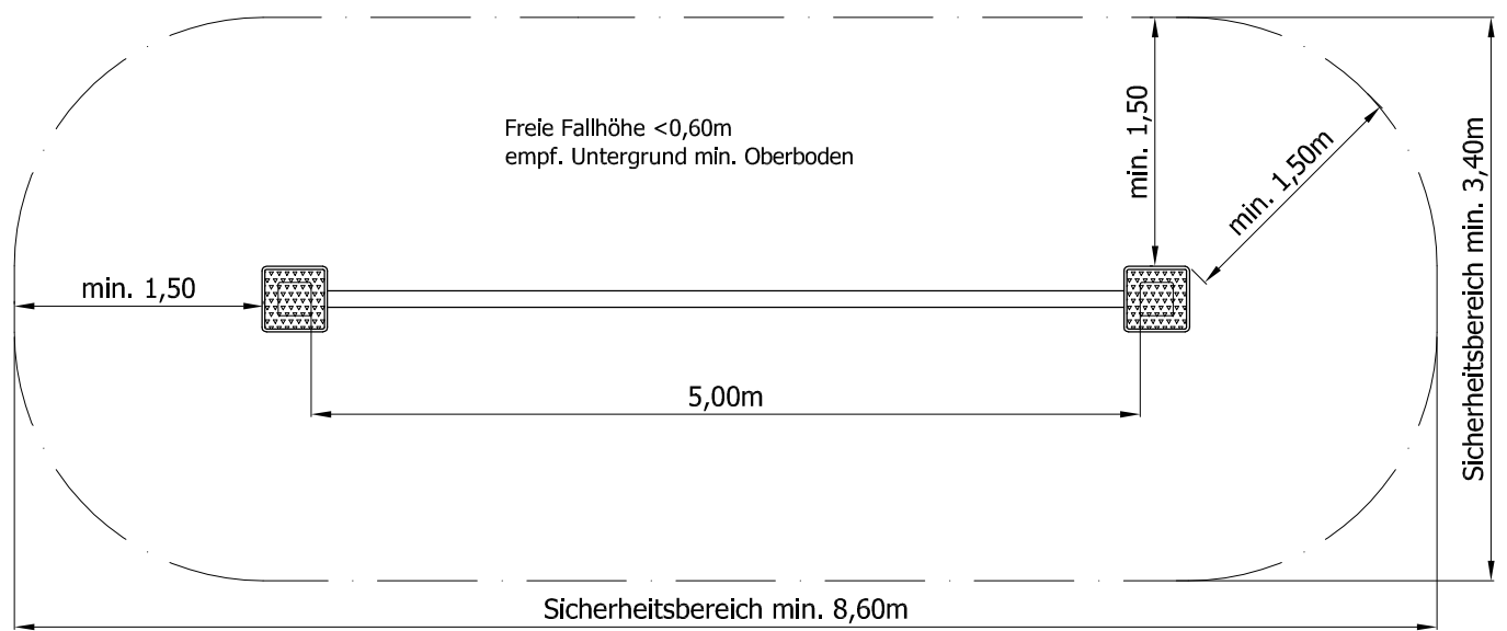
Draufsicht
