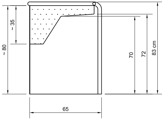
Seitenansicht Unterfahrbarer Sandspieltisch freistehend Art.- Nr.: 09 6070E
