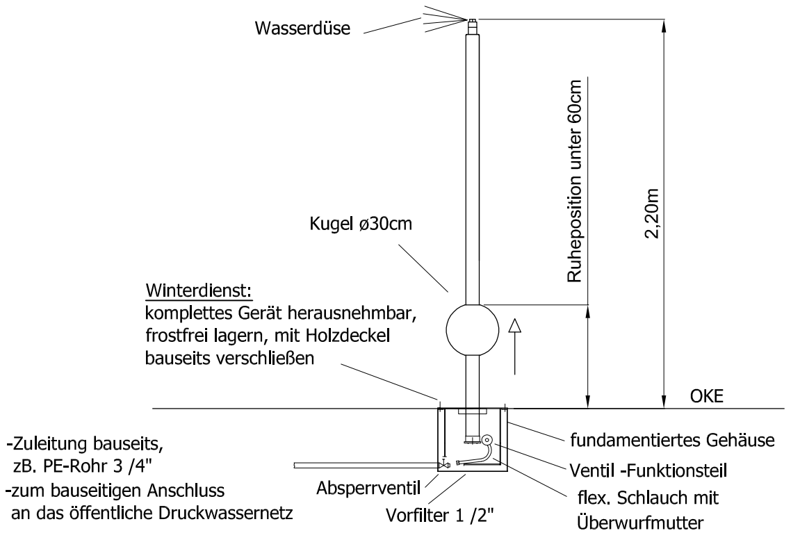
Ansicht
