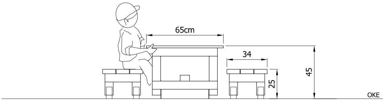
Ansicht -M -1:20-
