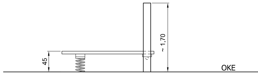
Ansicht
