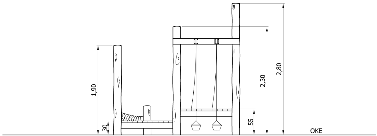
Ansicht
