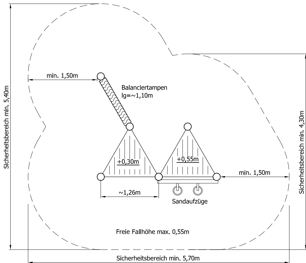
Draufsicht
