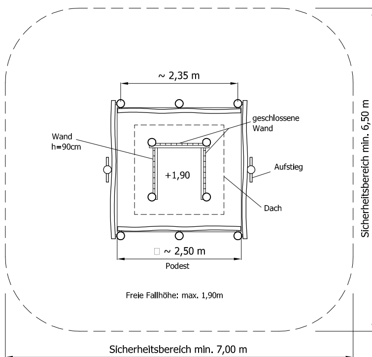
DRAUFSICHT
