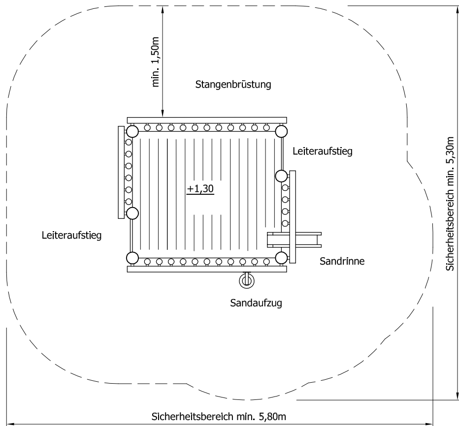
Draufsicht
