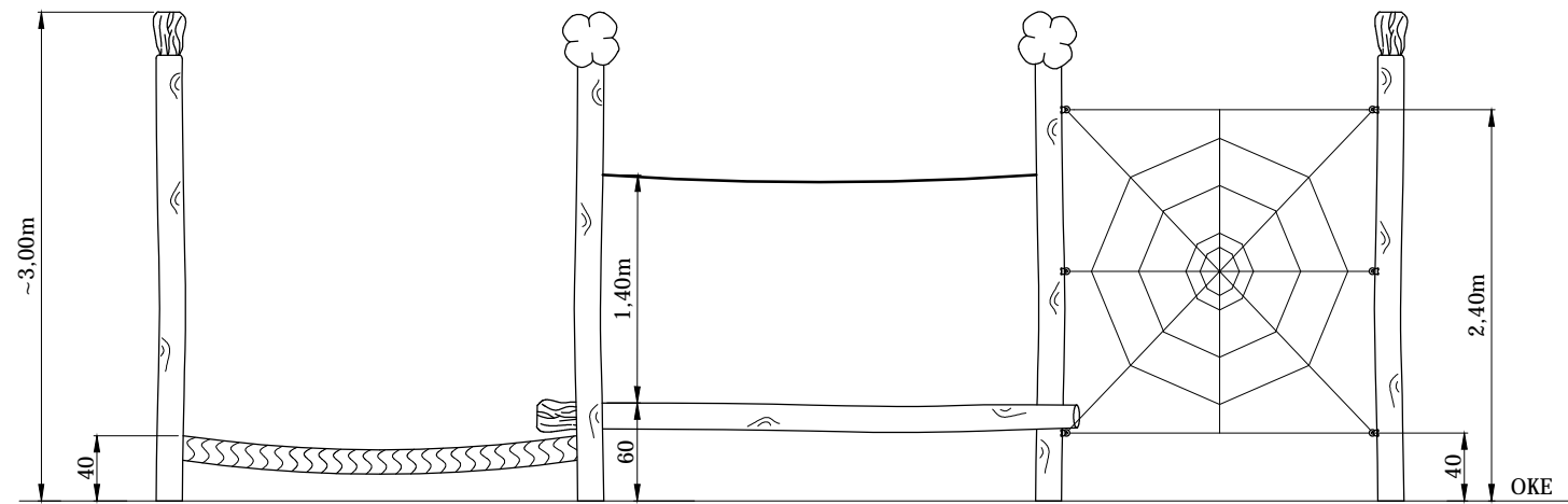
Ansicht
