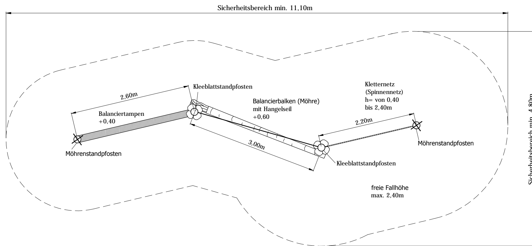
Draufsicht
