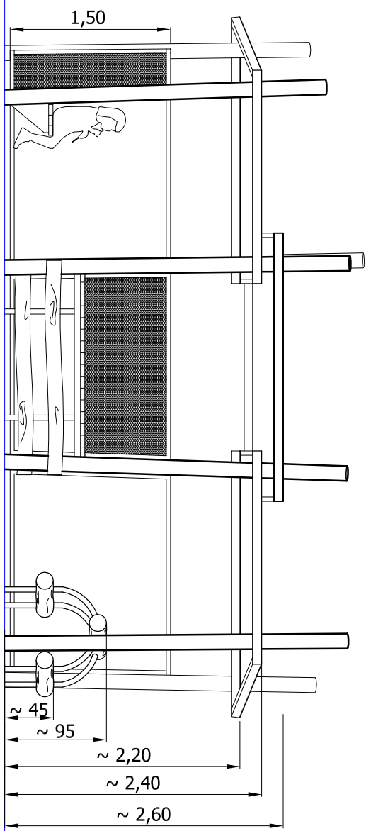
Ansicht OKE
