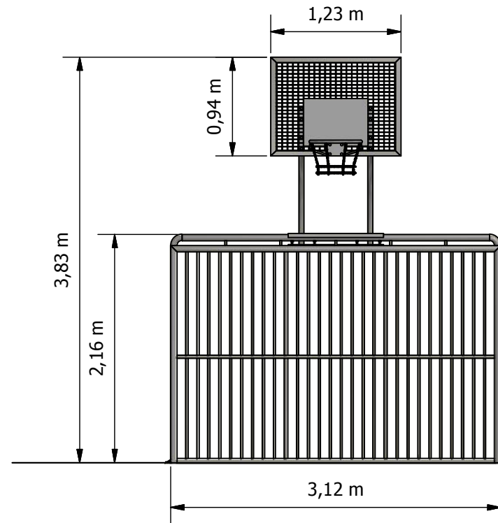
Vorderansicht ( 1 : 50 )
