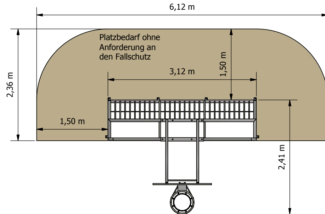
Draufsicht ( 1 : 50 )
