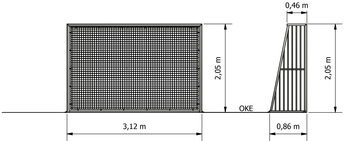
Seitenansicht ( 1 : 50 )
