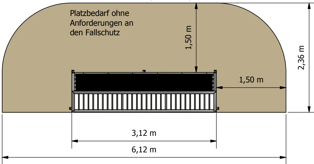
Draufsicht ( 1 : 50 )
