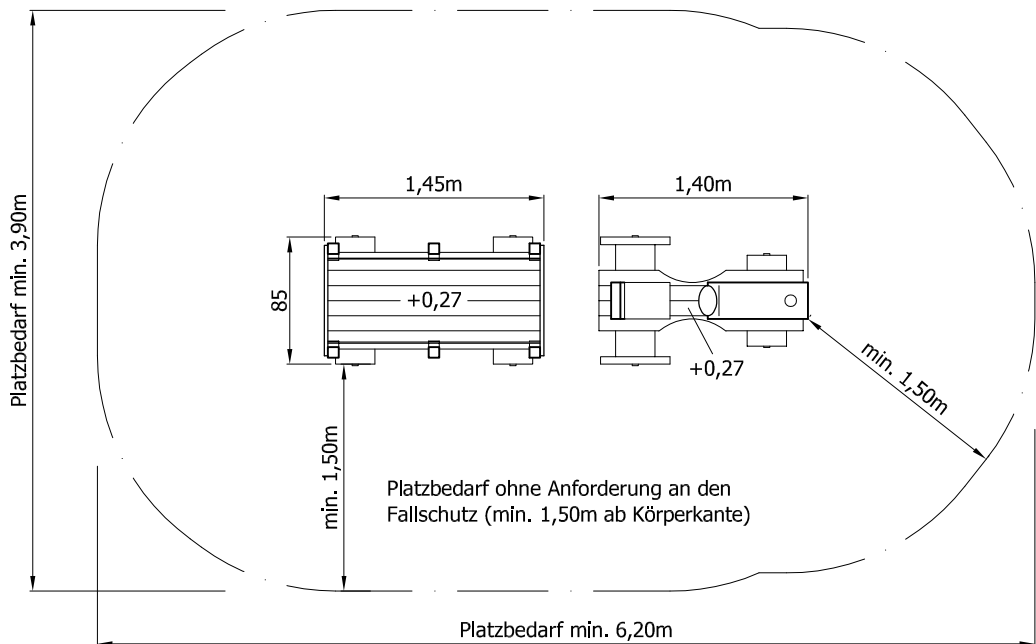
Draufsicht -M. 1:50-
