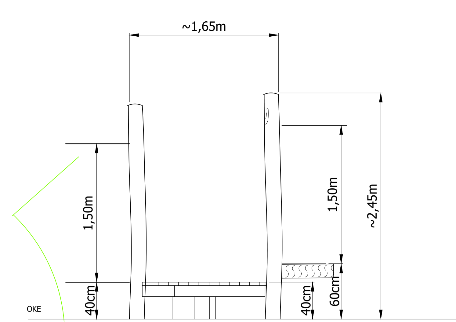
ANSICHT -M1:25-
