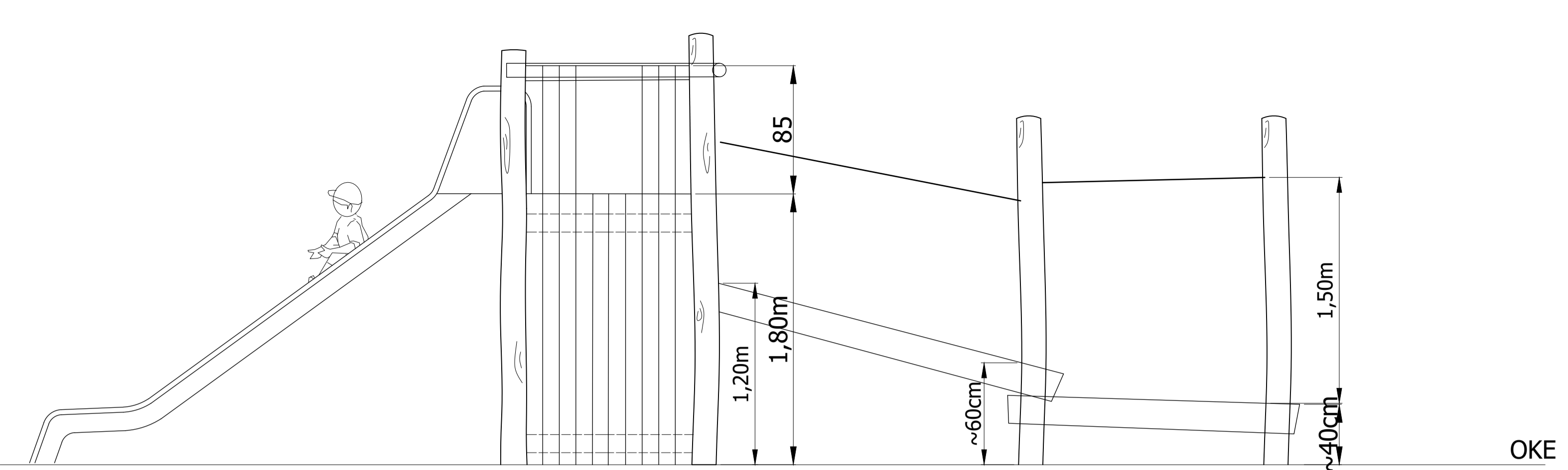
ANSICHT von links -M1:25-
