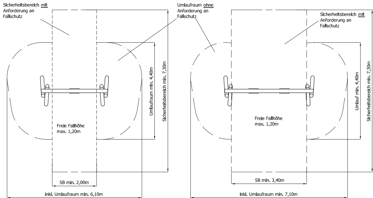
Draufsichten
