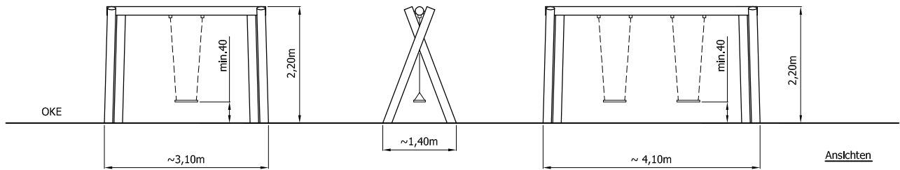
Kleine Einzelschaukel Art.-Nr.: 02 2901D/R (Einzellager)
