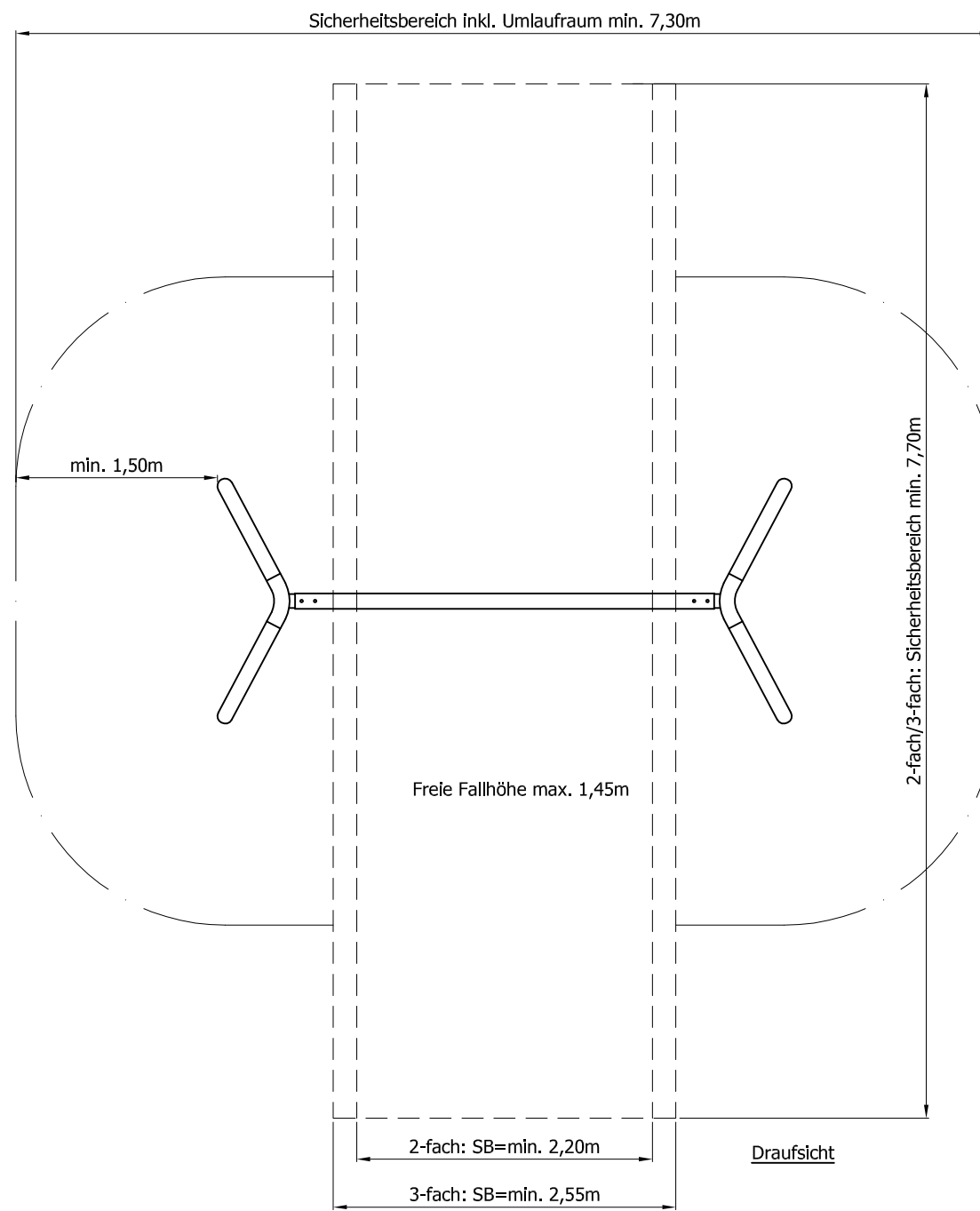
Ausführungsbeispiel
