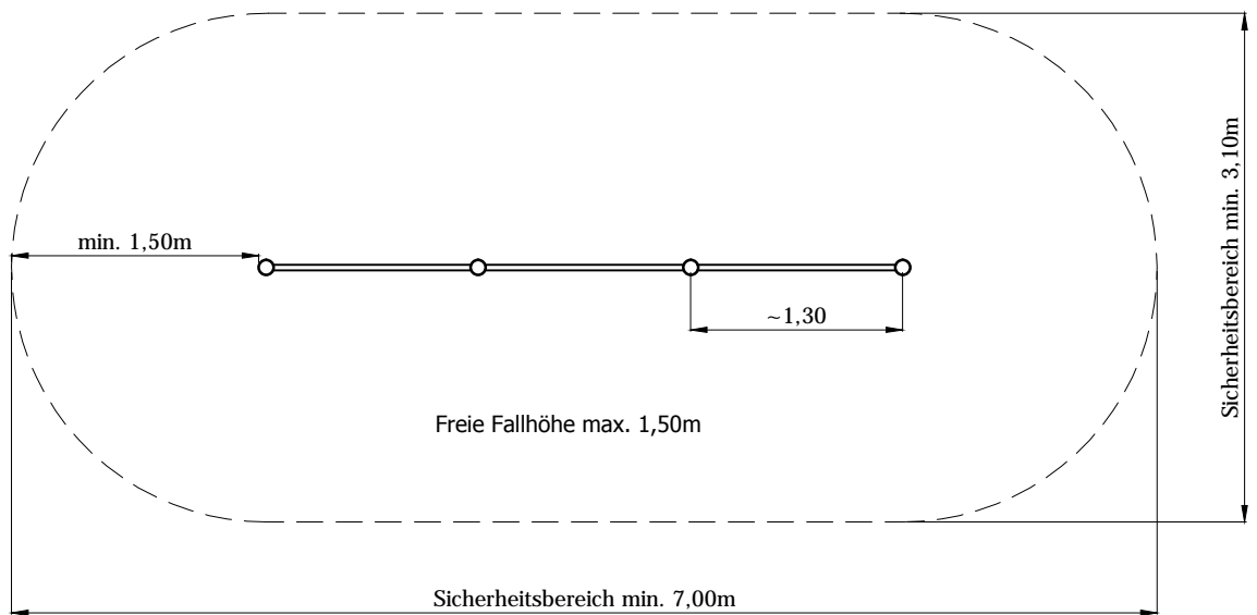
Draufsicht
