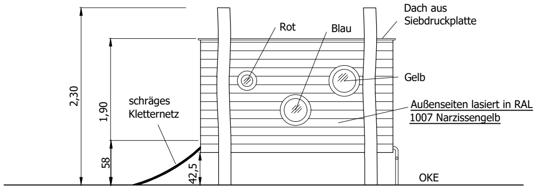
Ansicht
