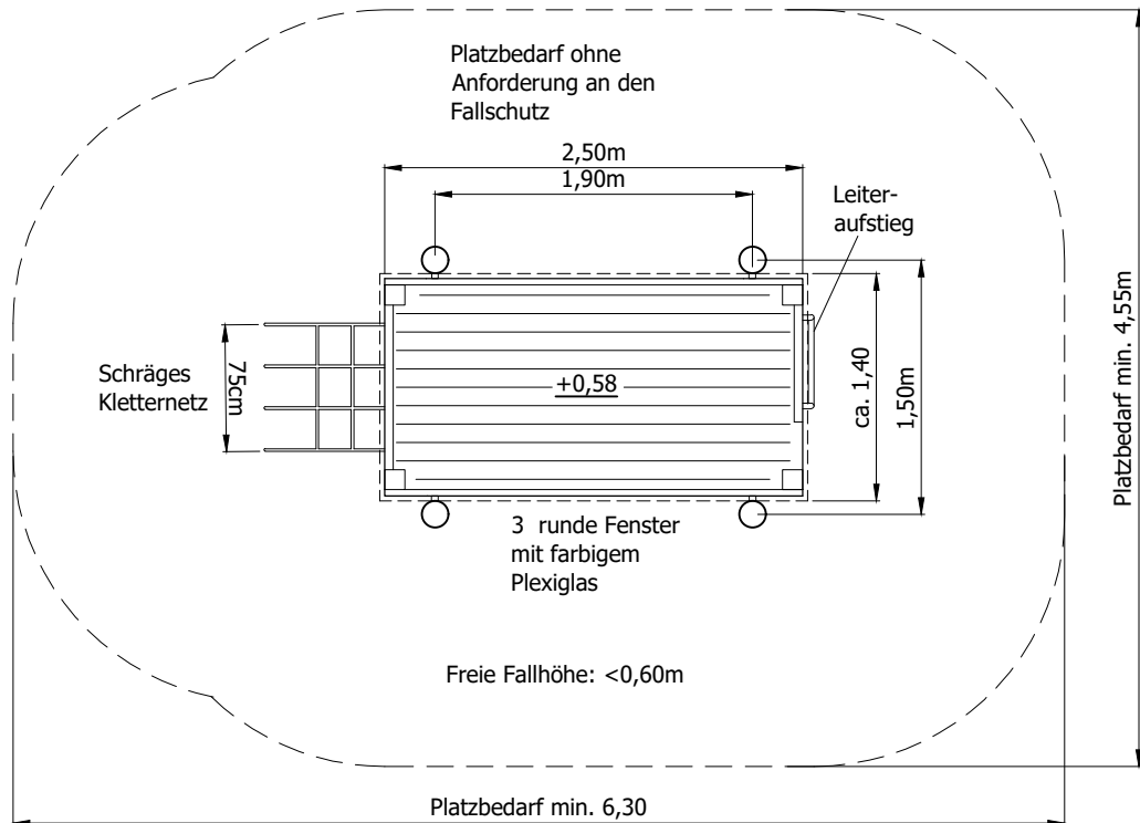
Draufsicht
