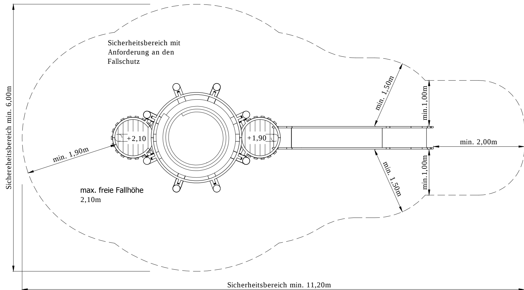
Draufsicht M-1:50-
