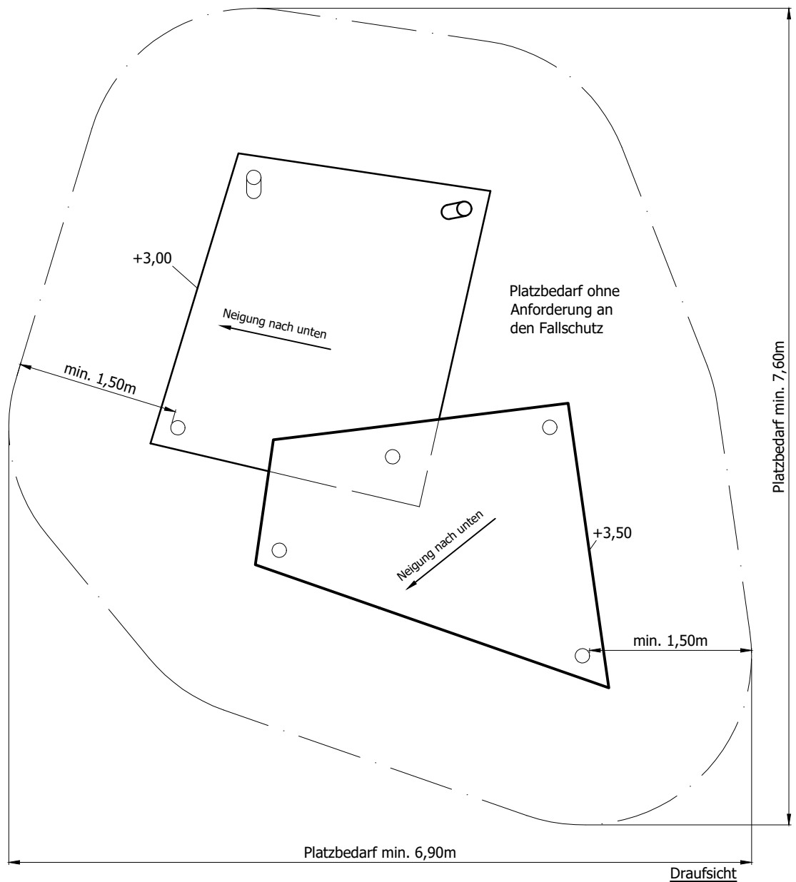
Draufsicht
